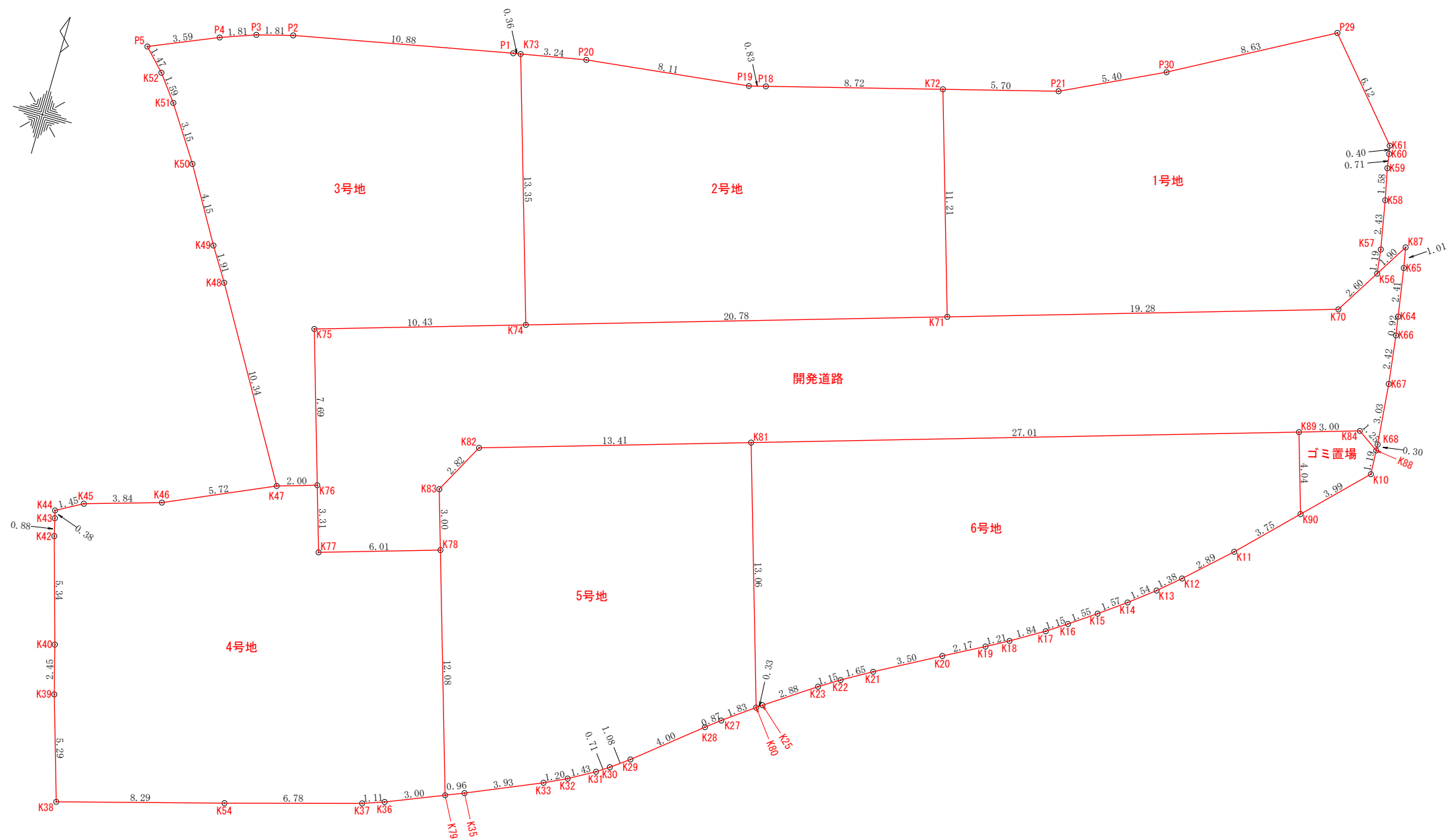
座標求積表
